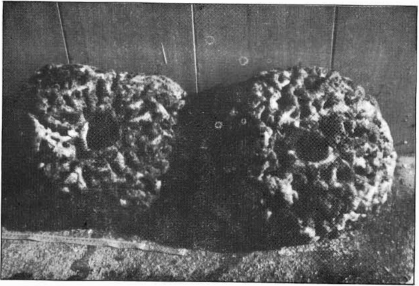
Fig. 1 - Due campioni dell'ecofenotipo di Geodia cydonium .
