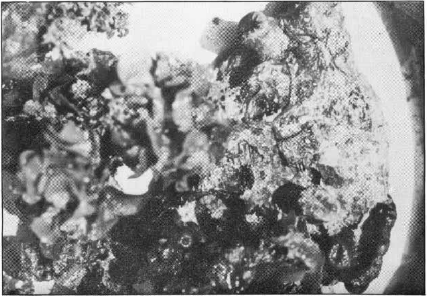
Fig. 3 - Agglomerato di Anadiomene stellata con Poriferi e Antozoi, inglobante fusti di Cystoseira .
